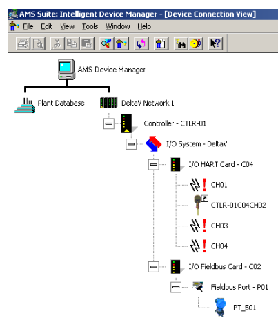
Afbeelding 1.1: DCS met instrumenten
